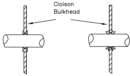
Dessin / Drawing N° 253-2
